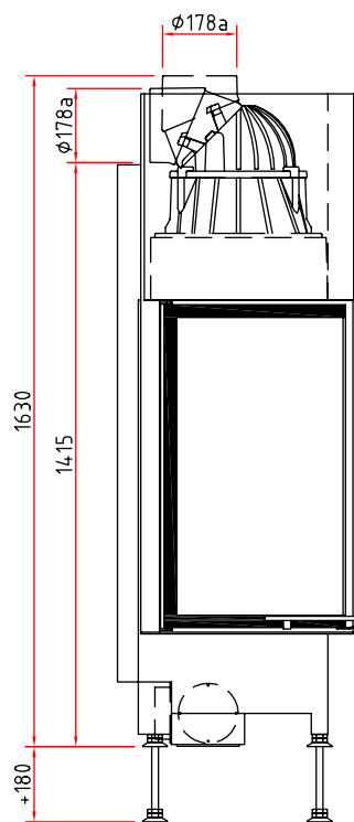
Vue de coté M 1:20
