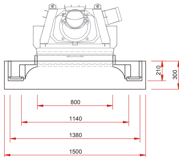
Draufsicht M 1:25
