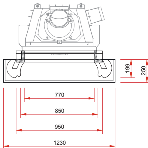
Draufsicht M 1:25
