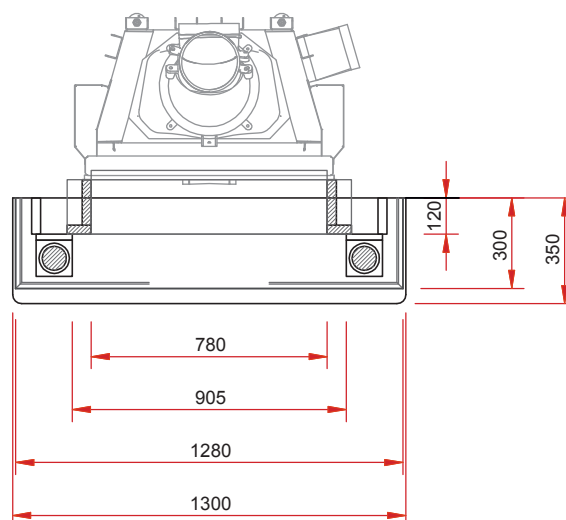
Draufsicht M 1:25
