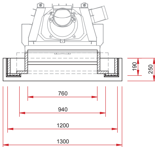
Draufsicht M 1:25
