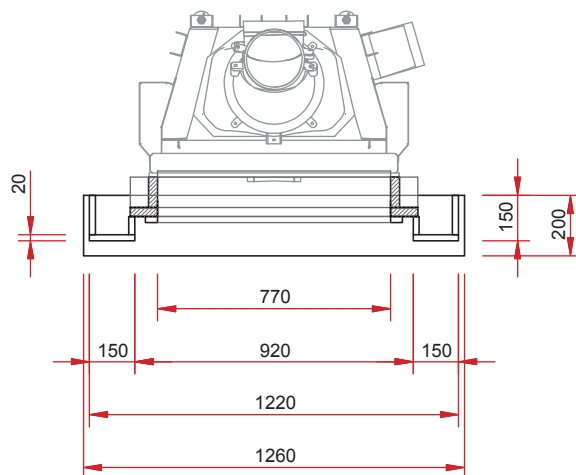
Draufsicht M 1:25
